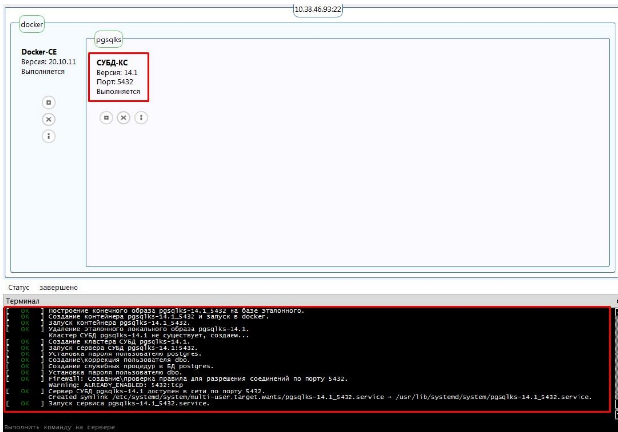
Рисунок 35. Лог установки контейнера «СУБД-КС Docker»
